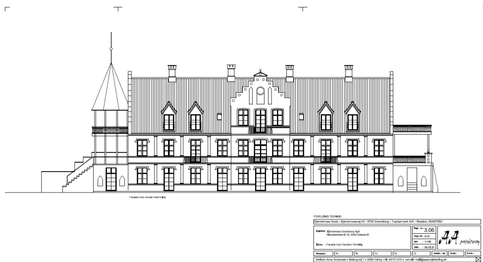
Fig. 2b. Facadetegning fra ansøgningen, der viser facade mod syd (vandsiden) efter genopførelse.
