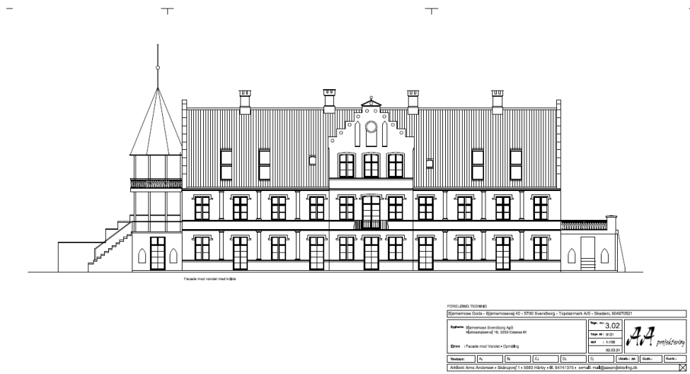
Fig. 2a. Facadetegning fra ansøgningen, der viser facade mod syd (vandsiden) før branden.
