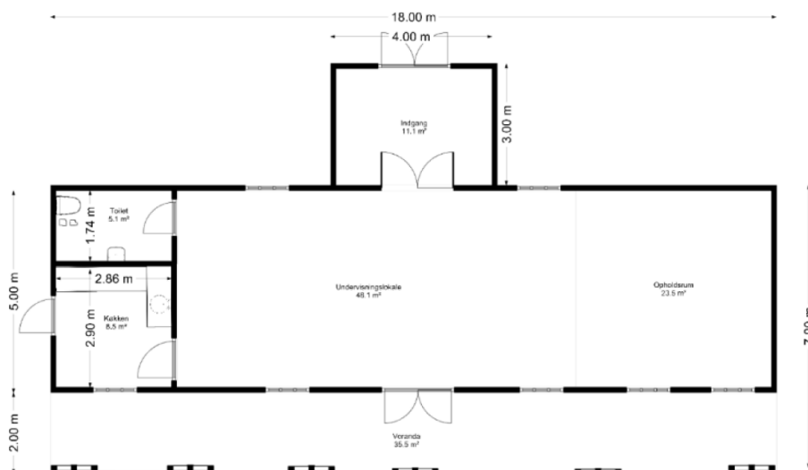
Fig. 4. Grundplan for den ansøgte natur- og friluftshytte.
