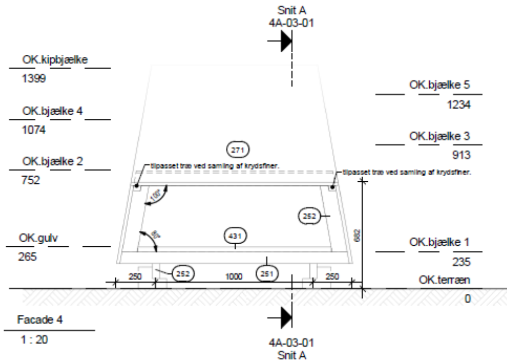
Facadetegning af shelteret Skrubben med mål.
