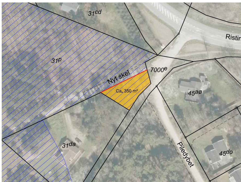
Gult område arealoverføres til offentlig vej 7000e. Rød linje nyt skel
