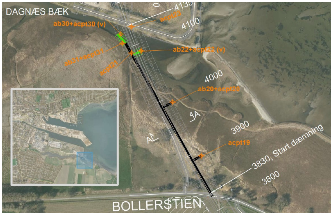
Figur 1 - Oversigtskort med undersøgelsespunkter (orange), midlertidige køreveje og arbejdsplanum på land (sort) og i bækken (grøn) samt den planlagte del af den nye ringvej (grå). Stationering er angivet i meter.
