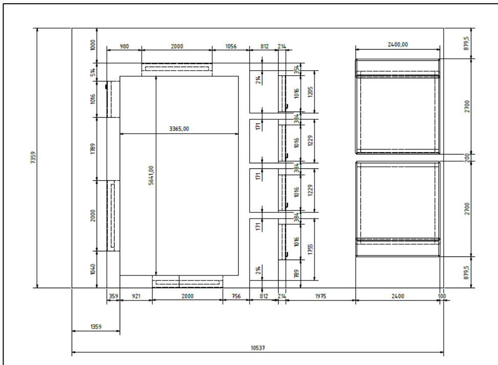
Fig. 3. Grundplan for det ansøgte. Shelters ses til højre. Havnebassinnet ligger mod venstre på tegningen, således at de to shelters placeres mellem bygningen, der indeholder klubhus og skoven.
