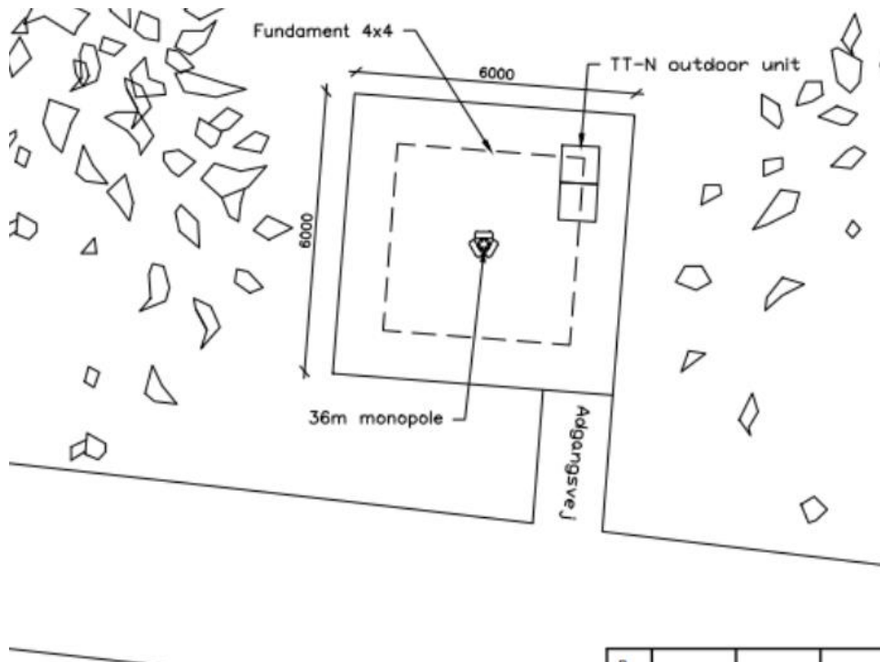
Figur 3: Plantegning af målene på fundamentet og mastens højde.
