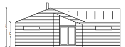
Facade mod nord/vest
