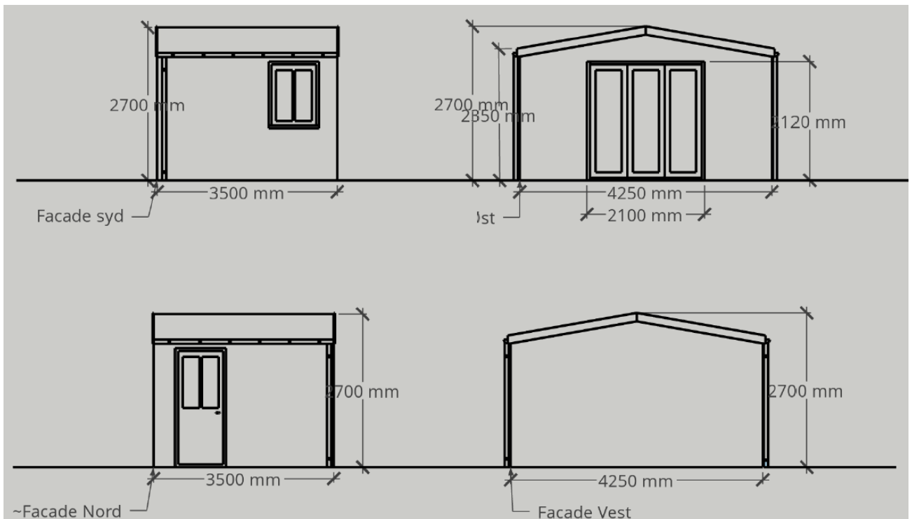
Medsendt skitsetegning over det ansøgte skur
