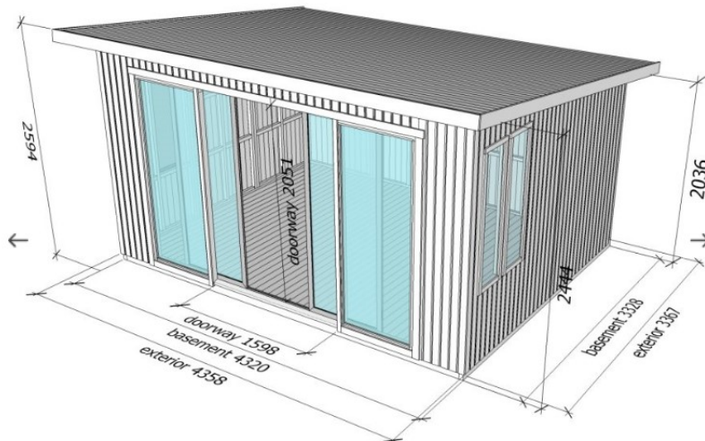
Taget er sort og uden vinduer – højden er 2,6 m mod vandet
