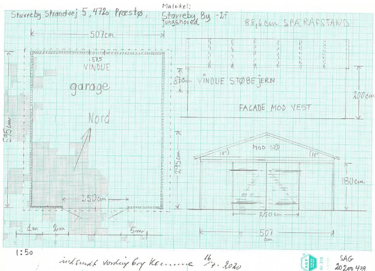
Fig. 3. Skitse af den ansøgte carport.
