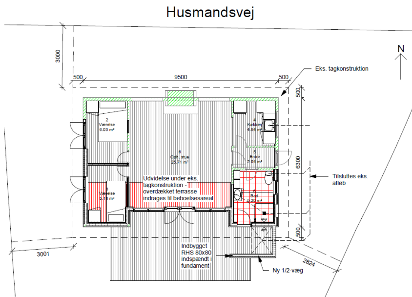
Figur 3, projekttegning fra ansøgning
