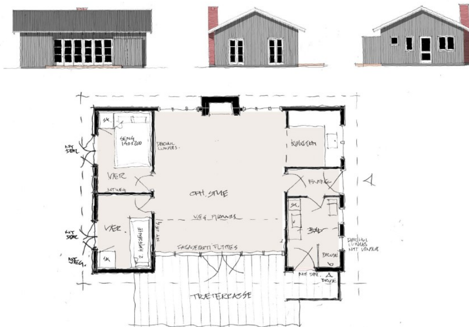
Figur 2, plan og facader fra ansøgning
