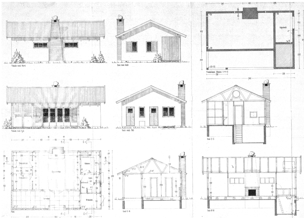
Figur 1, tegning af eksisterende hus, fra ansøgningen
