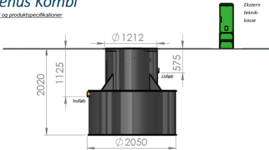
Figur 3. Tegning fra ansøgningen, der viser eksempel på minirenselanlægget, dækselstørrelse og teknikkasse.
