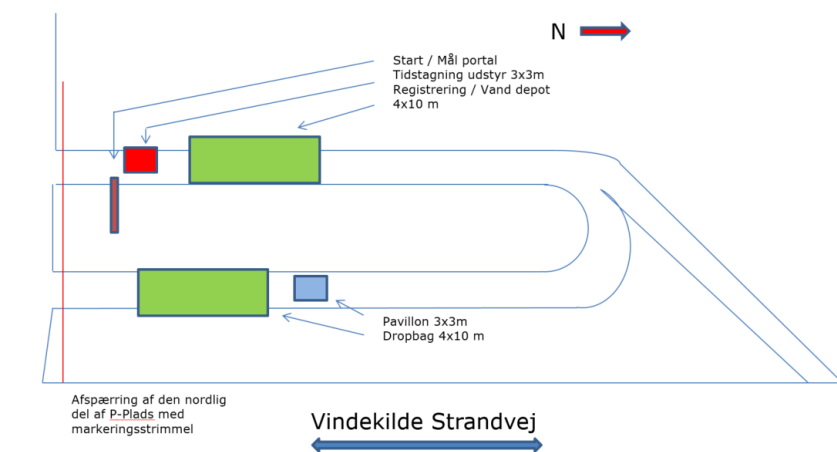
Vejrhøj Familie Trail 2020 COVID-19 opsætning Situationsplan for opsætning af telte, pavilloner og andre konstruktioner.
