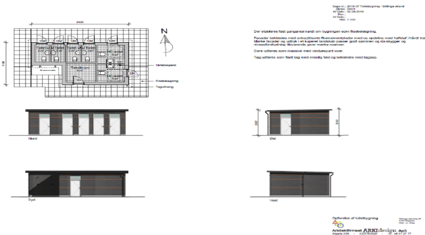
Figur 4. Facadebeklædning og teknisk tegning af toiletbygningen
