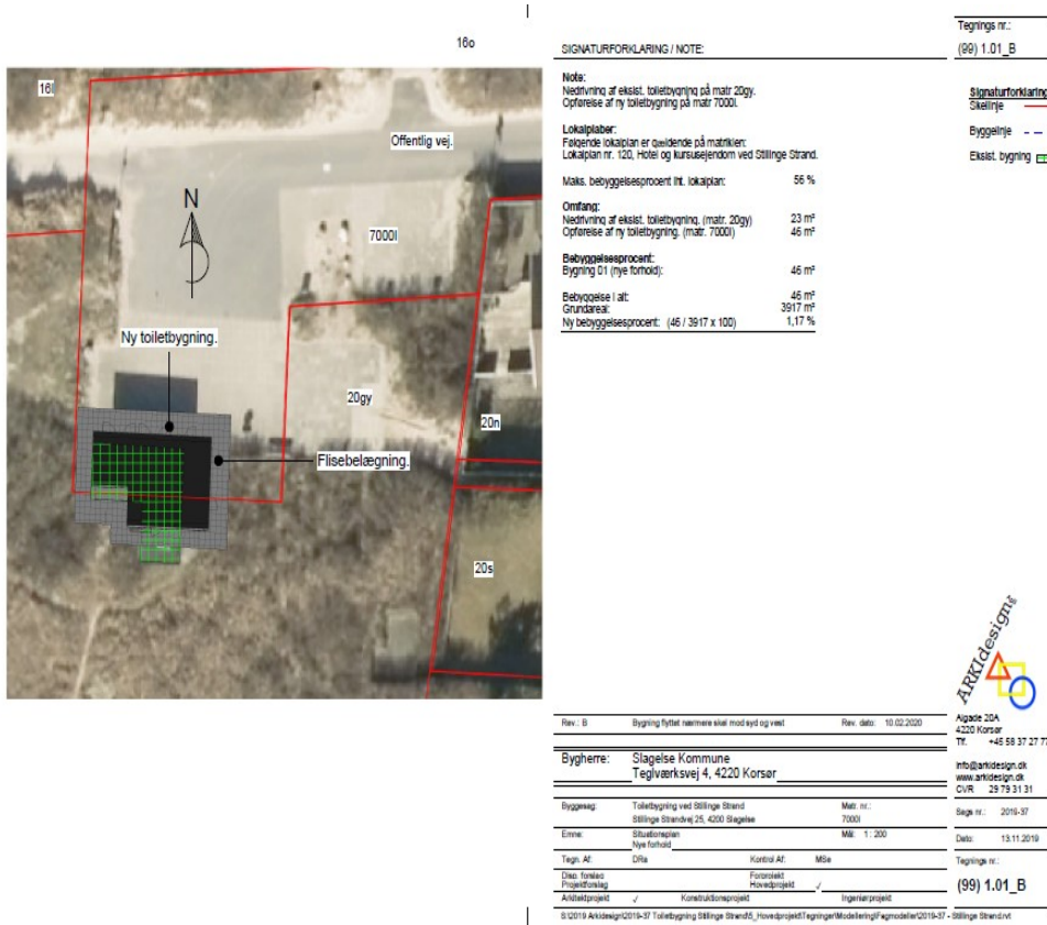
Figur 3. Placering af ny og eksisterende toiletbygning. Flisebelægning er markeret med gråt og eksisterende toiletbygning er vist med grøn skravering.
