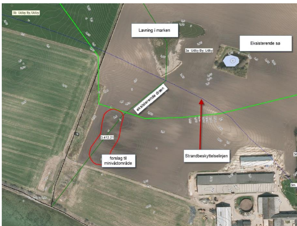
Fig. 2. Figur fra ansøgningsmaterialet, der viser placeringen og konstruktionen af det ansøgte minivådområde.
