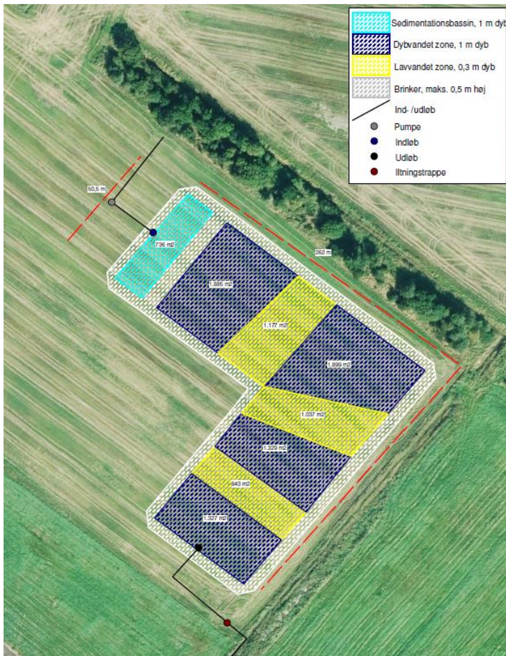
Fig. 2. Figur fra ansøgningsmaterialet, der viser placeringen og konstruktionen af det ansøgte minivådområde.
