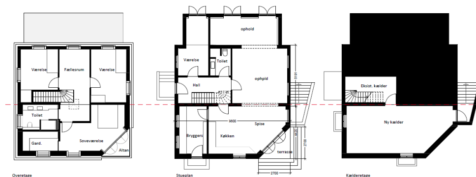
Figur 2. Plantegning fra ansøgningen, der viser hovedhuset og tilbygningen efter genopførelse.
