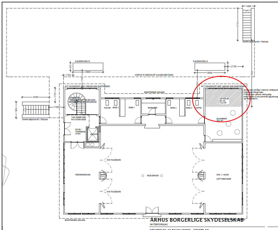
Skitse af bygningen i stueplan indsat fra ansøgningen. Udvidelsen på 12 kvm er markeret med rød. Øverst ses et rids af kælderen, kældertrapperne og ovenlysvinduerne.
