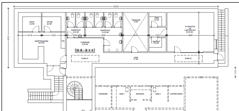
Skitsering af den søgte kælder. Ovenlysvinduer er markeret som stiplede rektangler. Kældertrapperne ses øverst til højre og nederst til venstre.
