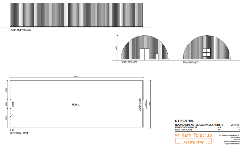
Figur 2. Tegning fra ansøgningen, der viser ridehallens størrelse og udformning.
