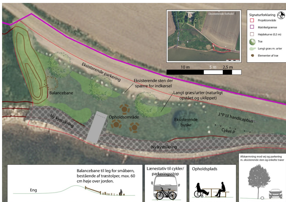
Fig. 3. Illustrationsplan for det ønskede på Rærup Strand/Peterspladsen. Grå firkant der går igennem kystsikringen illustrerer rampen.
