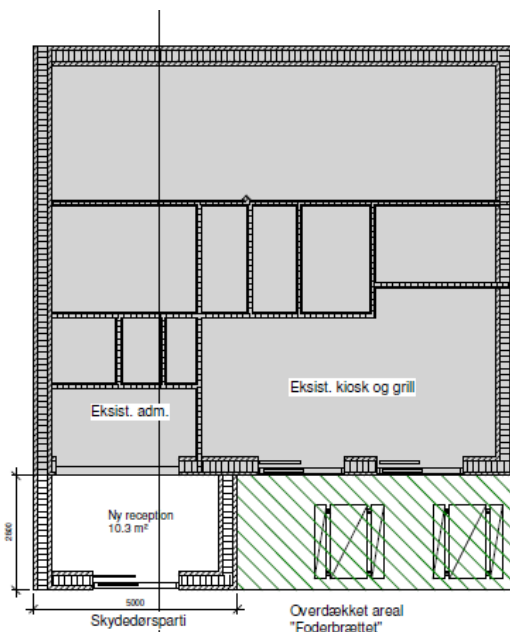
Plantegning af tilbygning, fra ansøgning
