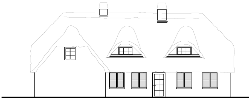
Tegning der viser den nye facade mod syd. Indsendt af ansøger.
