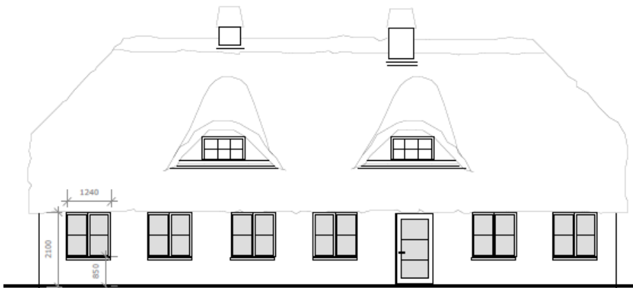
Tegning der viser den nye facade mod nord. Indsendt af ansøger.
