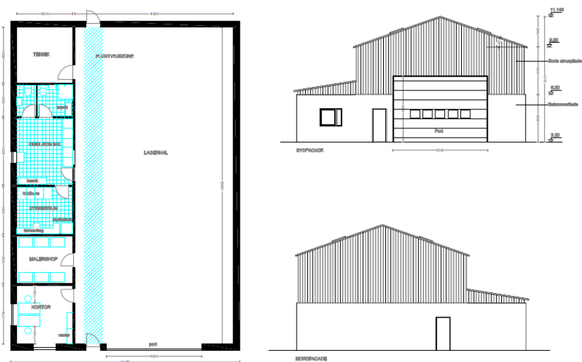
Fig. 3. Plantegning af erstatningsbygning samt nord og syd facaden.
