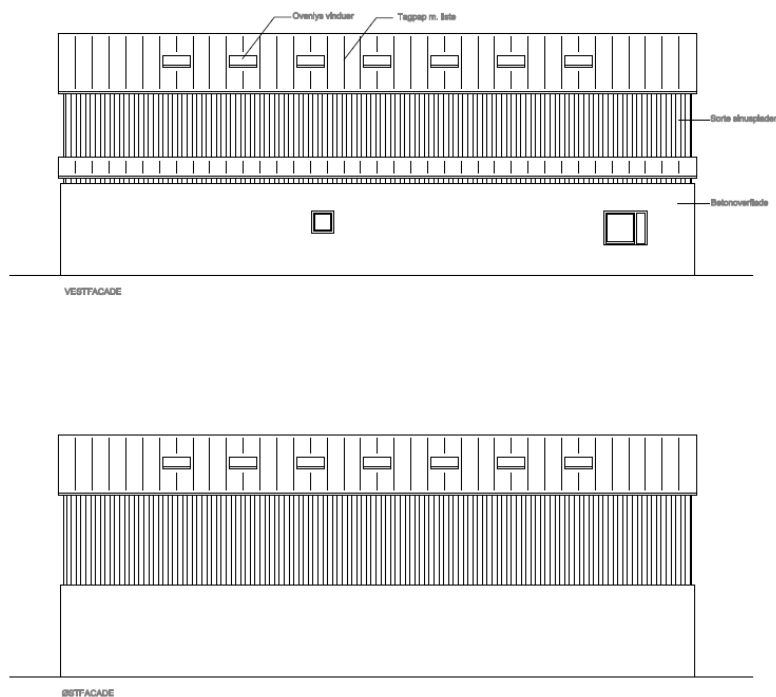
Fig. 4. Øst og vest facaden af erstatningsbygning.
