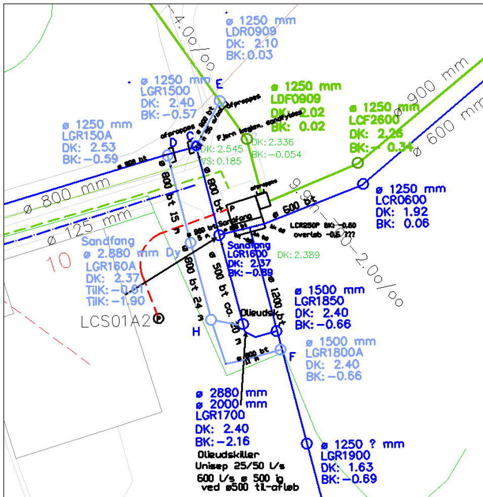
Figur 2. Illustration af forholdene efter projektet er gennemført. Regnvand omdirigeres igennem ny ledning som etableres parallelt med den eksisterende via fire nye brønde markeret med lyseblå cirkler og bogstaverne E, D, H og F.
