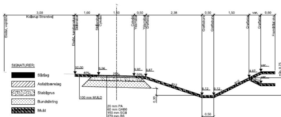
Fig. 4. Tværsnit af den ønskede cykelsti og afvandingskonstruktion.
