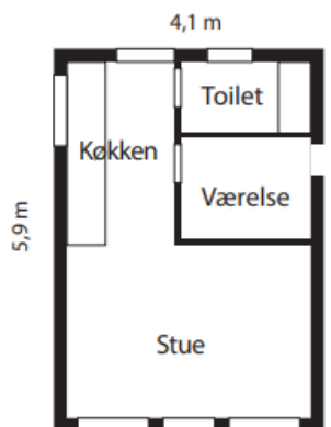
PLAN 1:100
