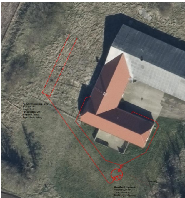
Siveanlæg og bundfældningstank med dæksler
