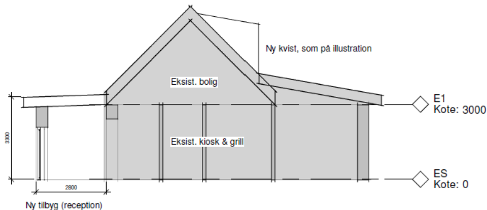
Tegning fra ansøgning, opstalt af reception, overdækning og kvist
