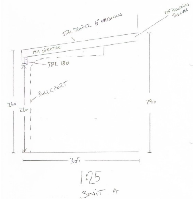
Figur 3, tegning af gavl, fra ansøgning
