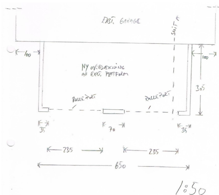
Figur 2, tegning af tilbygning, situationsplan fra ansøgning
