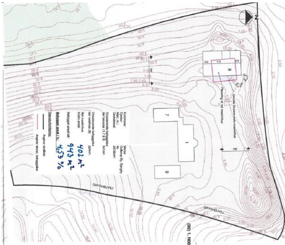
Figur 3: Situationsplan, hvor placering af nuværende maskinhus (rød stiple) og nyt maskinhus er vist
