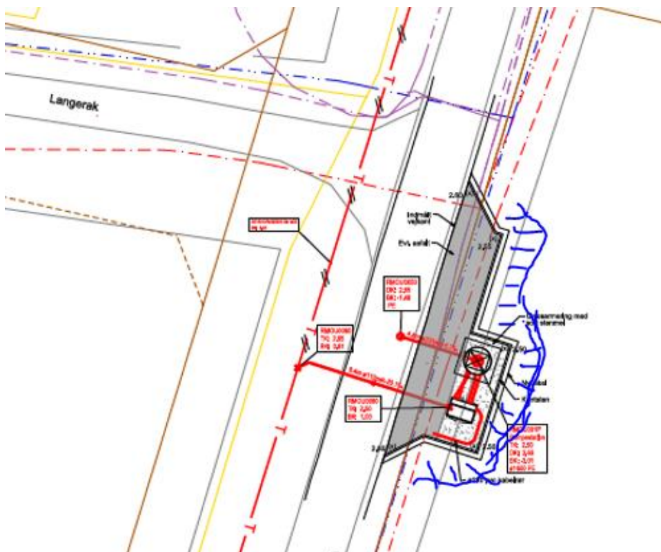
Vigeplads og anlæg af pumpestation etableres ved den blå markering. Under: Udstrækning af anlægget samt markering af areal for genplantning (blå).
