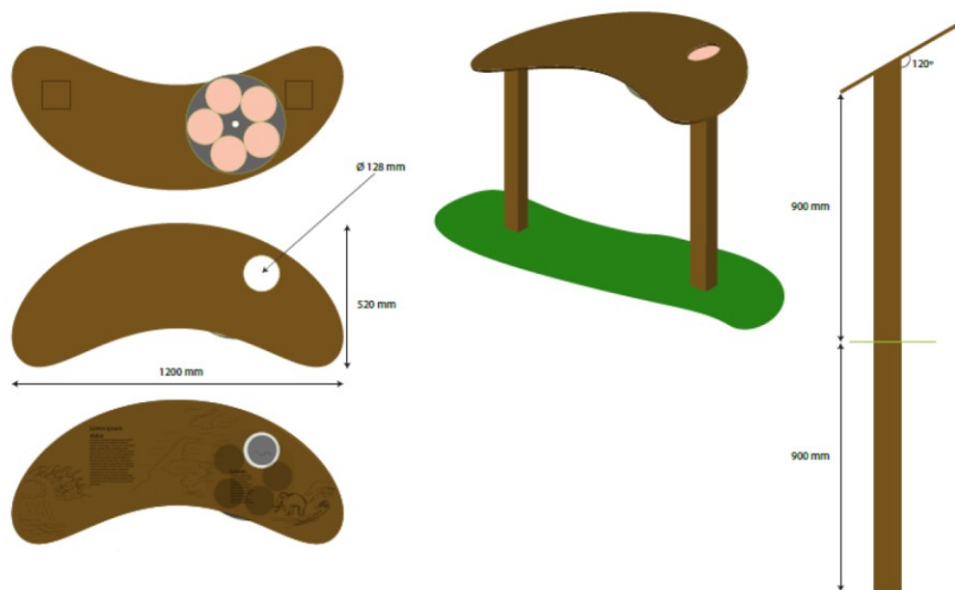
Figur 4: skitse over dimensioneringen af skiltene tilsendt af ansøger
