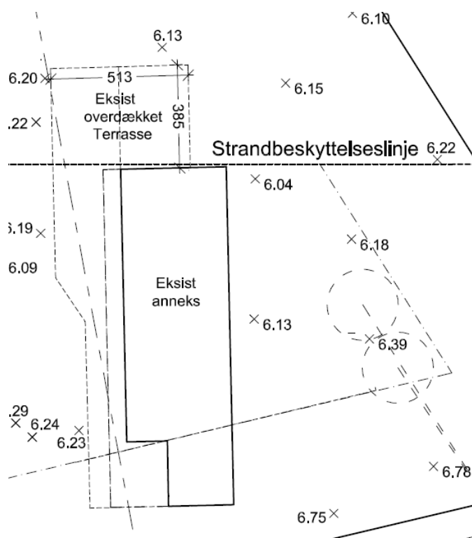
Figur 2. Indsendt af ansøger. Situationsplan der viser anneksets eksisterende terrasse og placering.
