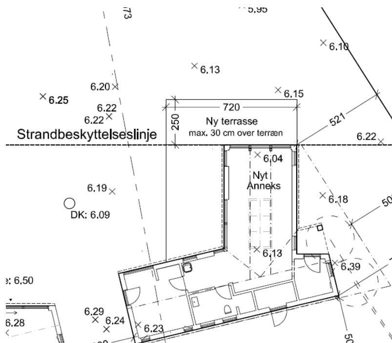
Figur 3. Indsendt af ansøger. Situationsplan der viser genopførelse af terrasse og annek.
