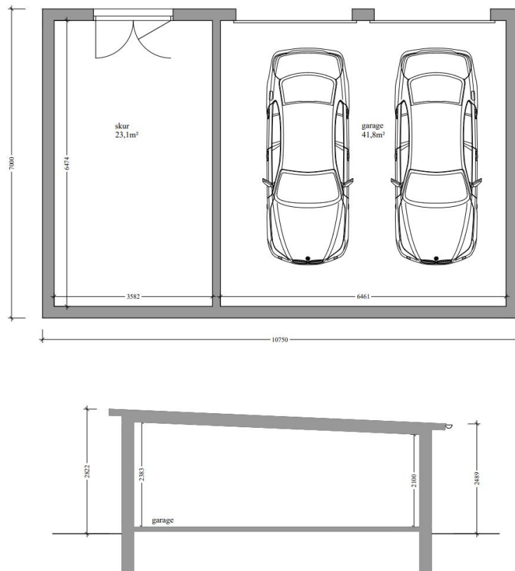
Fig. 2. Plan- og principsnit af garagen indsendt af ansøger.
