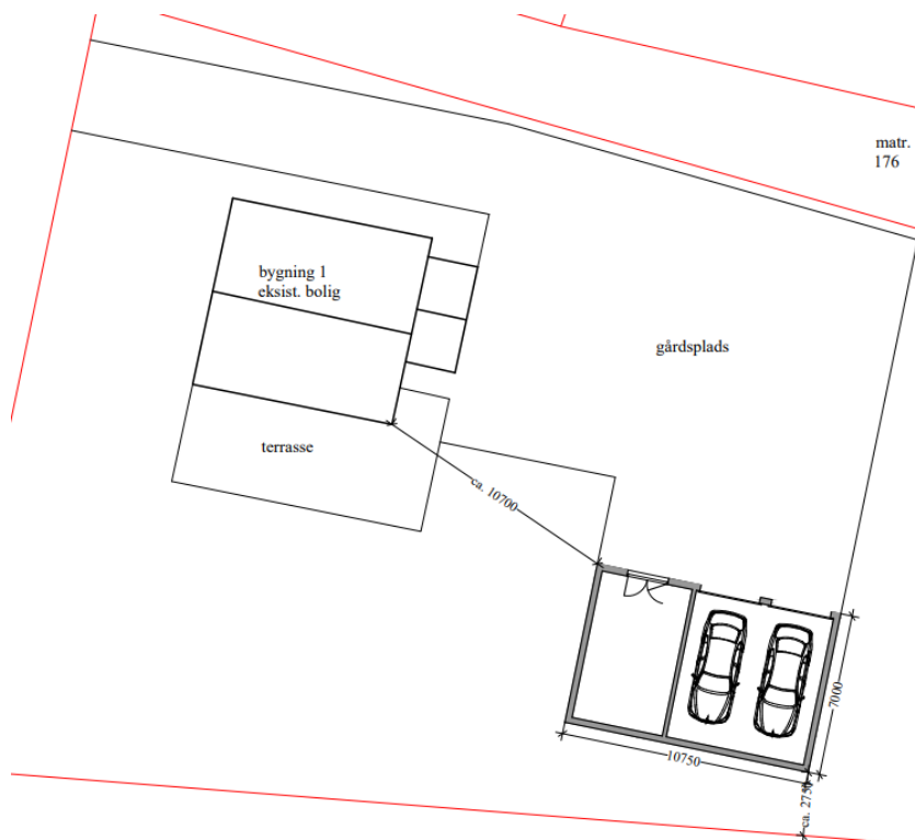
Fig. 3. Situationsplan over det ansøgte indsendt af ansøger.
