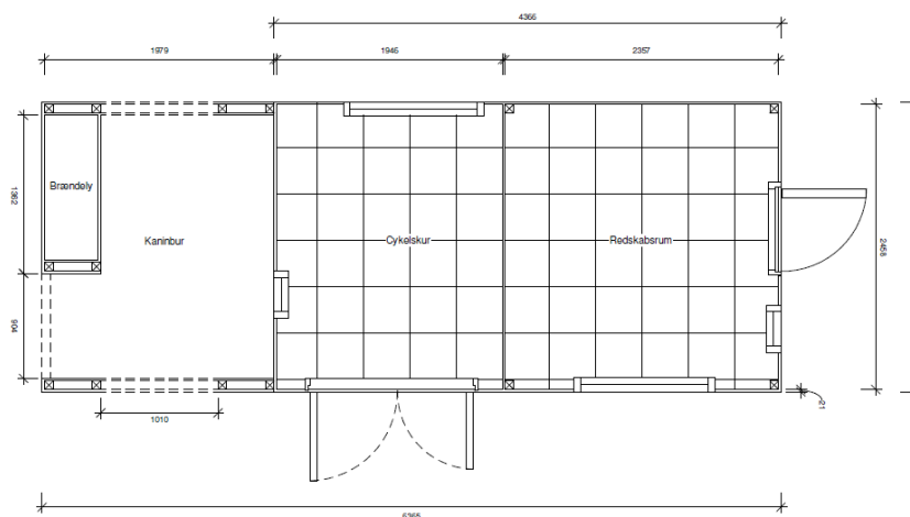
Fig. 9 viser plantegning over udhuset set fra venstre med brændely, kaninbur, cykelskur og redskabsrum. De samlede mål for udhuset bliver 6,4 m i længden og 2,5 i bredden hvilket giver 16kvm. Højden på huset med tag bliver ca. 2,3 m. Indsat fra ansøgning.
