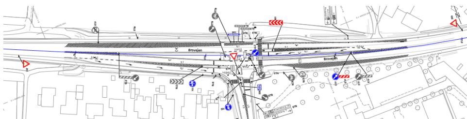
Afmærkningsplan
