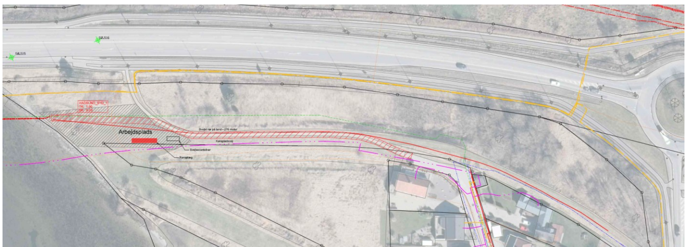
Fig. 3. Oversigtsplan over den midlertidige anlægsplads. Den gråskravering nærmest vandet er arbejdsarealet hvorpå der opsættes svejsecontainer og oplag af rør. Den røde skraverede linje viser udlæg af køreplader. Den røde linje der forløber fra vandet parallelt med vejen er det svejste rør på i alt 276 meter.
