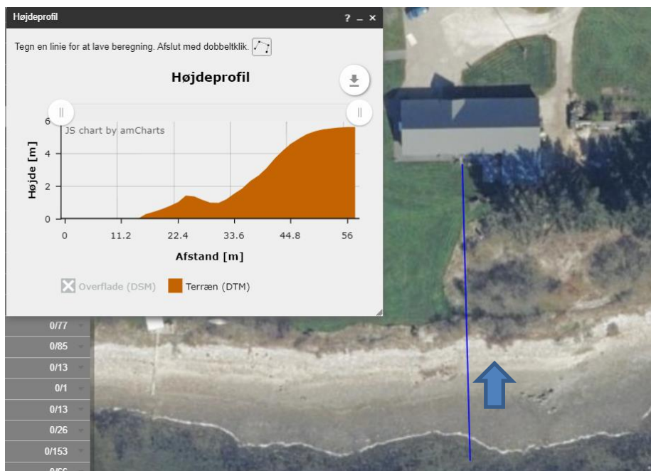
Fig. 2 Vejledende højdeprofil af terrænet. Den blå streg viser hvor målingen er sket og pilen viser retningen.
