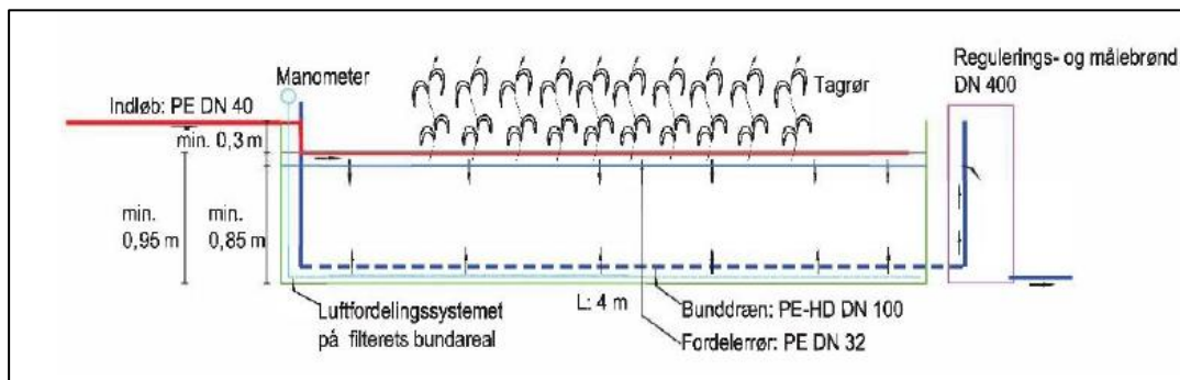
Principskitse af anlægget (snit)
