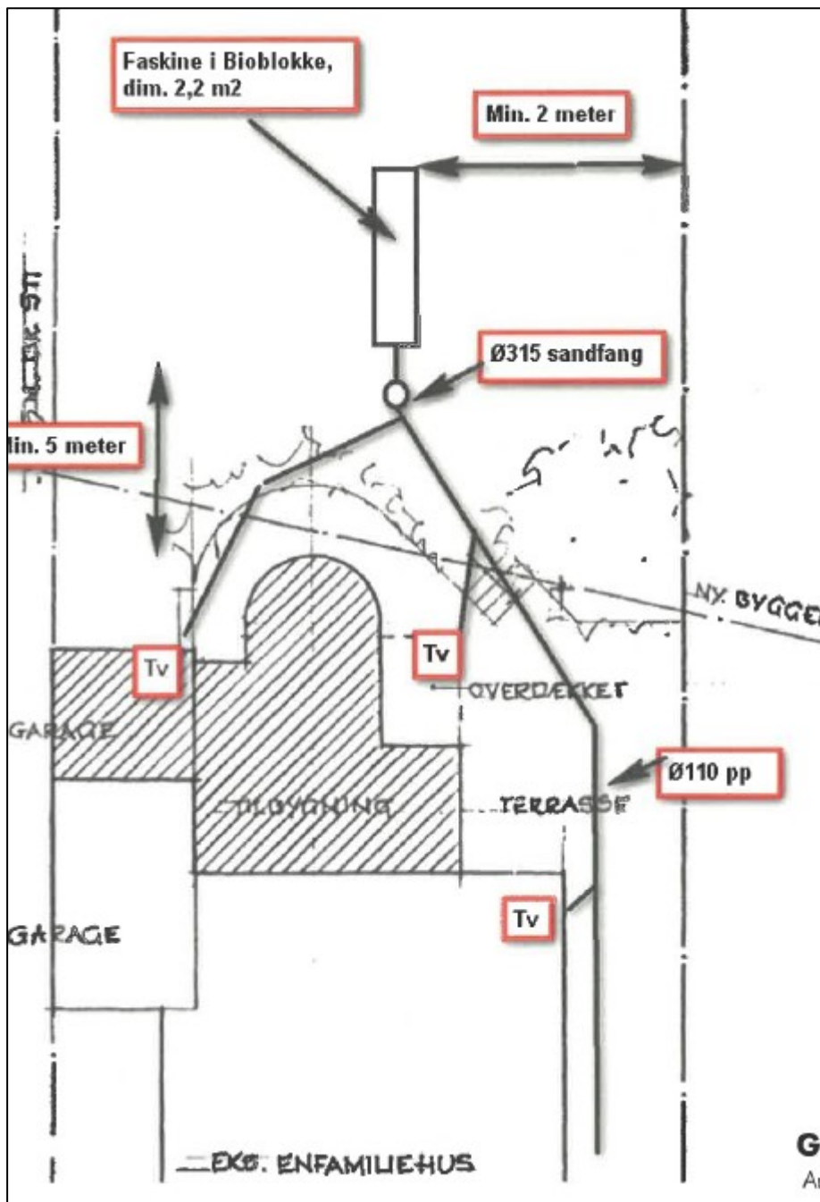
Situationsplan viser placering af faskine og brønd
