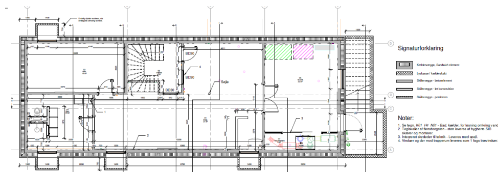
Kælderplan med udvendig trappe
