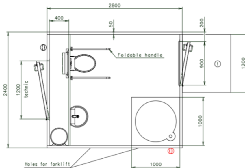
Fig. 3. Toiletbygningens mål og indretning (fra ansøgningsmaterialet)
