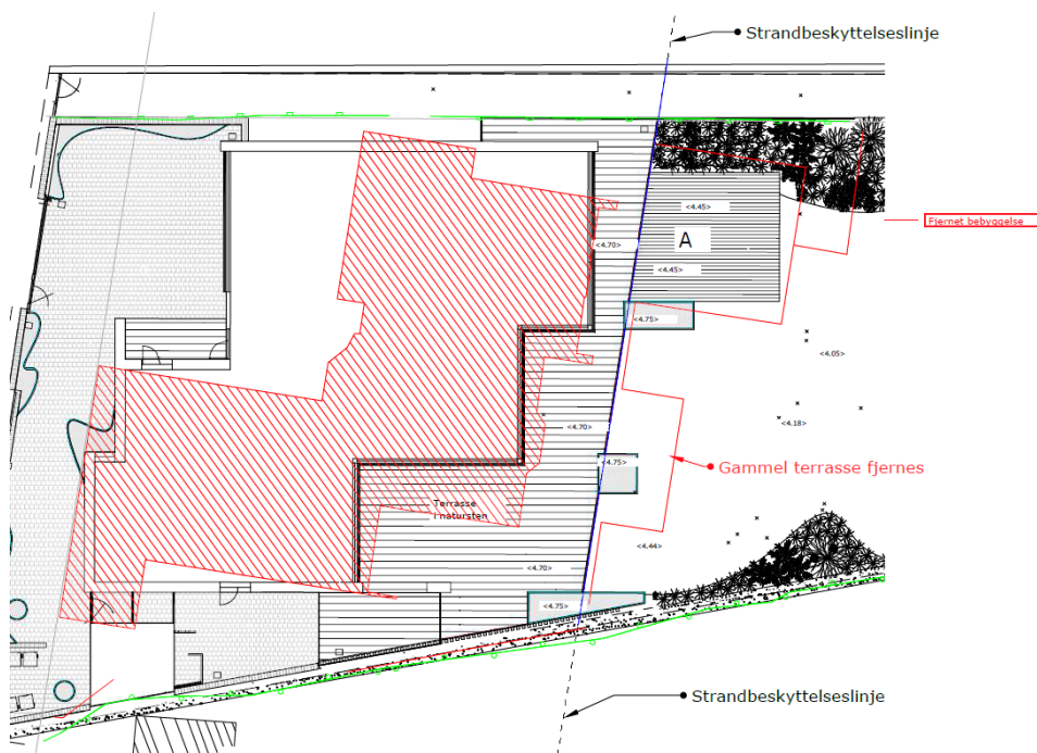
Fig. 3. Situationsplan vedlagt ansøgningen. Med rød skråskravering er vist beliggenheden af den tidligere bolig. Den røde linje inden for strandbeskyttelseslinjen viser en kantsten, der fjernes samt en gammel stenterrasse på ca. 15 m², der ligeledes fjernes.
