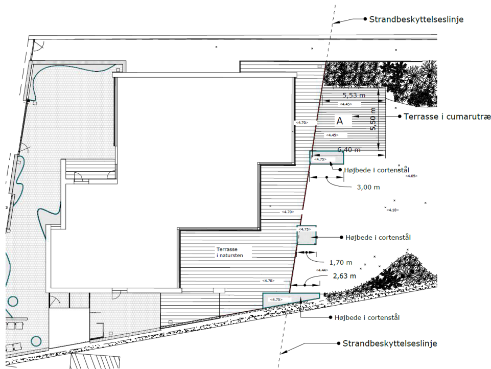
Fig. 2. Situationsplan vedlagt ansøgningen, der viser den ansøgte terrasse i cumarutræ samt højbede, der er undtaget fra kravet om dispensation, jf. § 15a, stk. 3.
