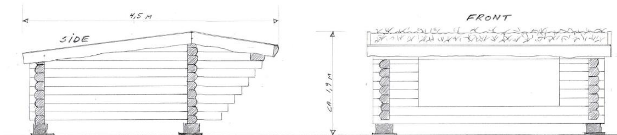
Figur 3 Fuldtømmer shelter model fi
