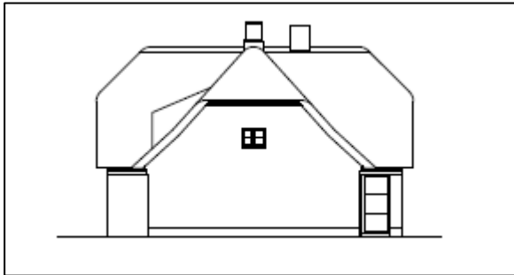
Facade mod vest, eksisterende forhold
