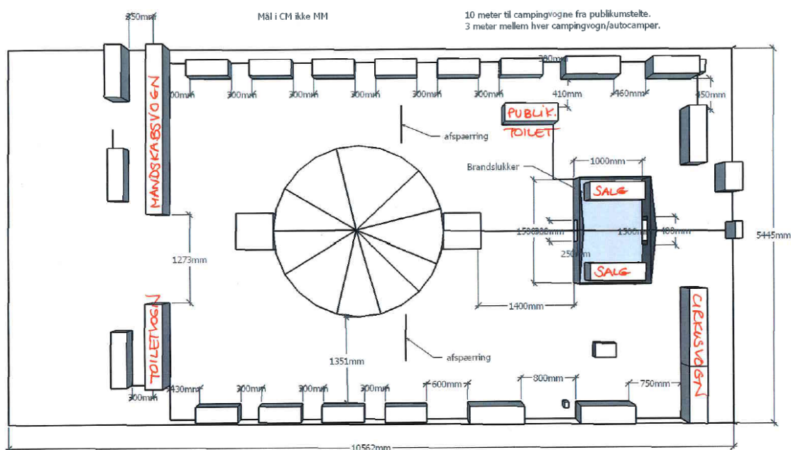
Situationsplan viser opstillingen. Indsat fra ansøgningsmaterialet.
