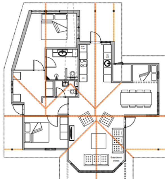
Ansøgt grundplan
