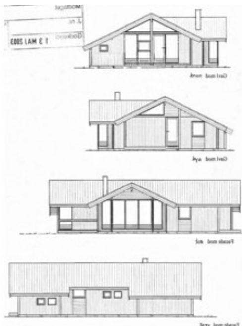
Eksisterende facader
