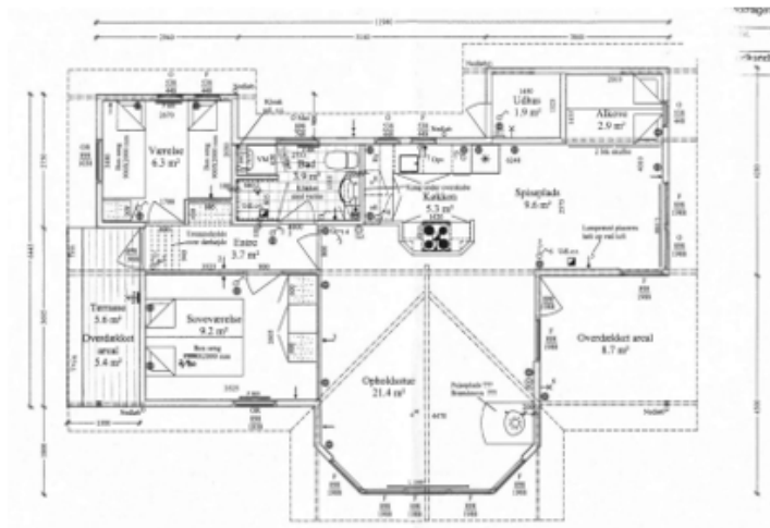
Eksisterende grundplan
