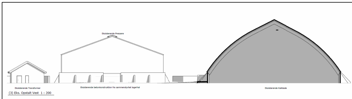
Opstalt set fra vest viser forholdene før bygningen styrtede sammen.
