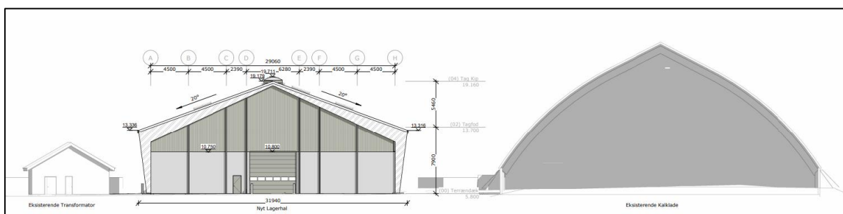
Opstalt viser ansøgte forhold.
