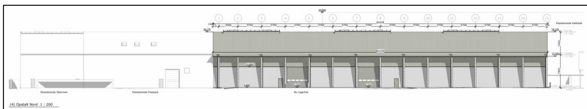
Opstalt viser ansøgte forhold. Facader md nord.
