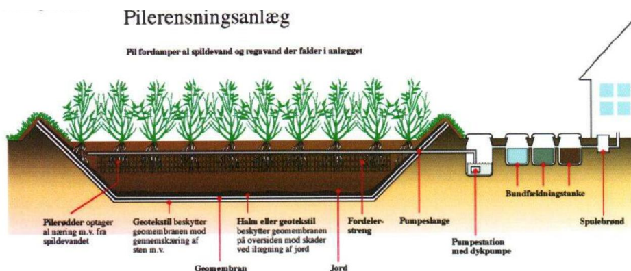
Fig. 4. Fra ansøgningsmaterialet. Snit af pilerenseanlæg
